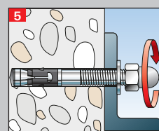
Hutmutter aufdrehen
